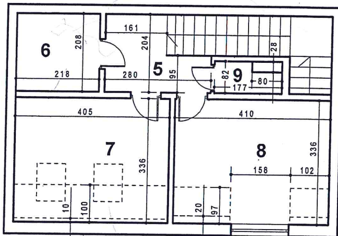
PODDASZE
