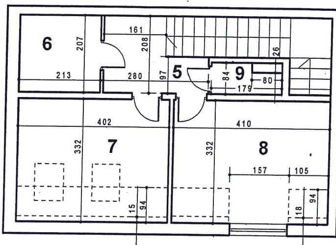
PODDASZE
