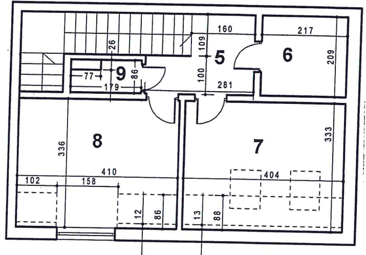
PODDASZE
