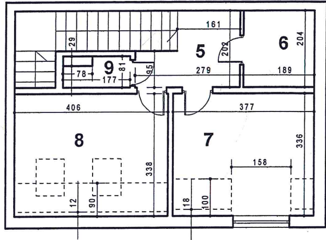
PODDASZE
