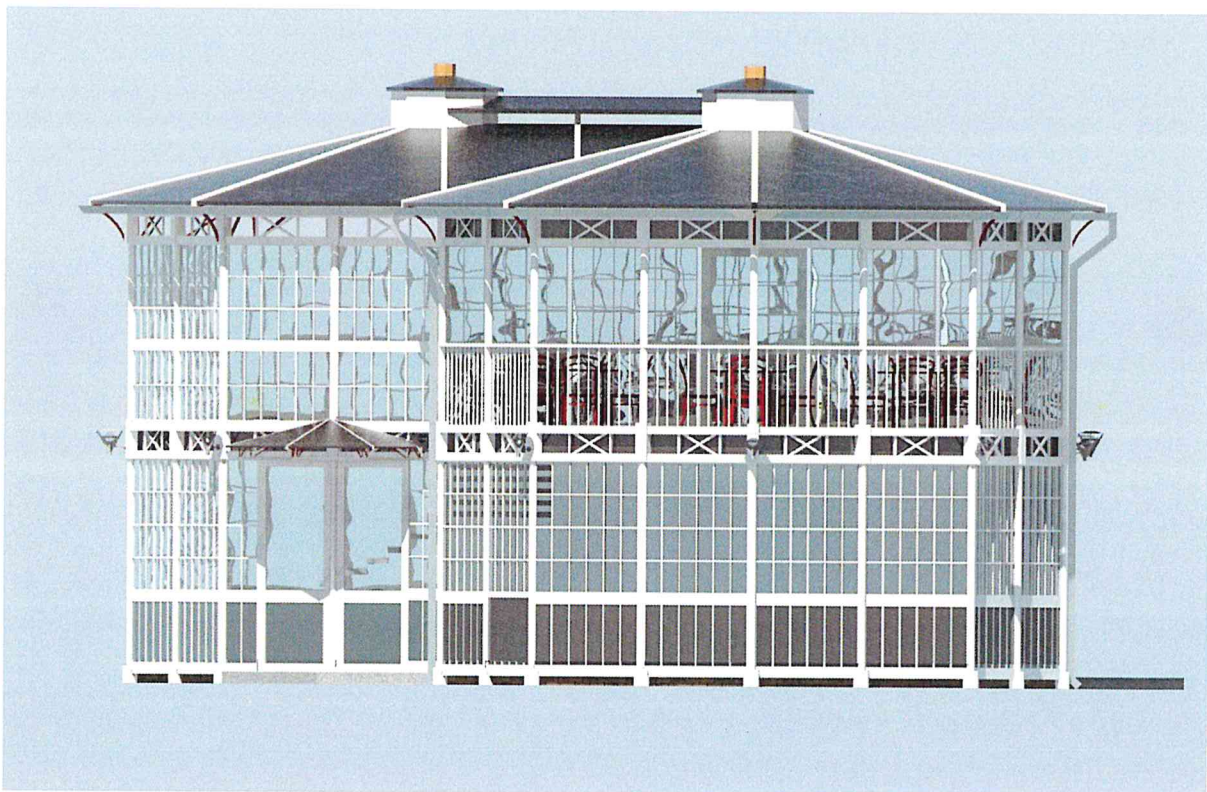
Elewacja szczytowa (południowa)
